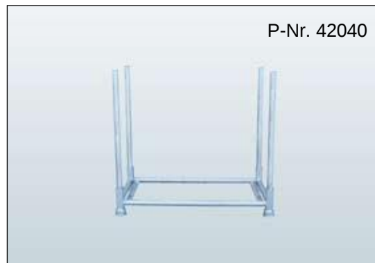
Bühnengitter Palette B/L/H: 83 x 1460 x 1310 mm, Gewicht: 41 kg
