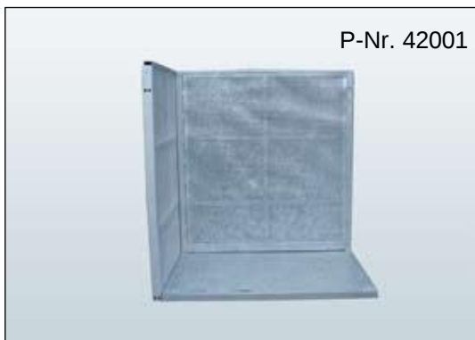
Bühnengitter 90° Vario-Kombi Typ S Innen/Außen: Oberes Rohr : 40x20 mm, Gewicht: 86,9 kg, Stahl
