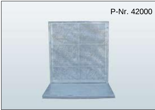
Bühnengitter Typ S · 1,19x1,10 m Oberes Rohr: 40 x 20 mm, Gewicht: 65,5 kg, Stahl
