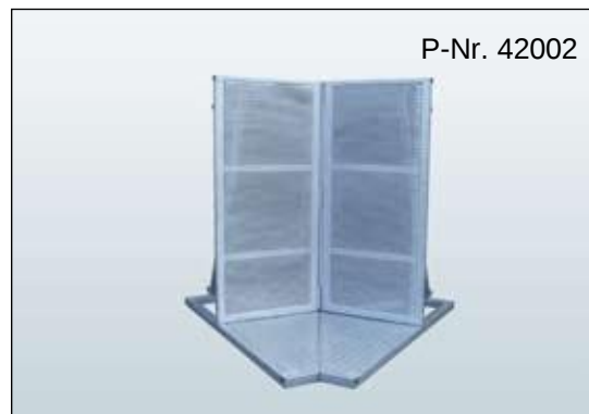
Bühnengitter 60° Vario-Kombi Typ S Innen/Außen: Oberes Rohr: 40 x 20 mm, Gewicht: 39,3 kg, Stahl
