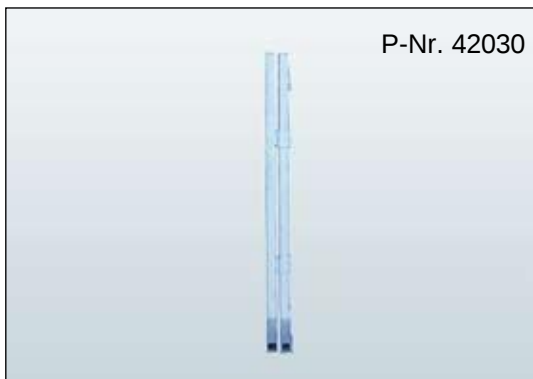
Bühnengitter Höhenausgleich Länge: 1190 mm, verstellbar bis Höhe 160 mm, Gewicht: 11,2 kg
