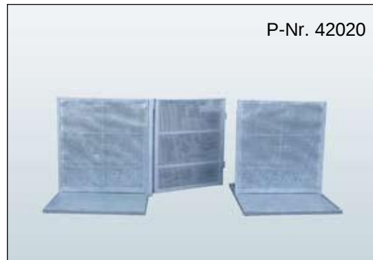
Bühnengitter Tür Typ S H/B: 1190 x 1050 mm, Oberes Rohr: 40 x 20 mm, Gewicht: 26,3 kg, Stahl
