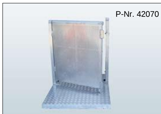
Bühnengitter Tür Typ A H/B: 1150 x 1000 mm, Oberes Rohr Ø 60 mm, Gewicht: 36,2 kg, Aluminium
