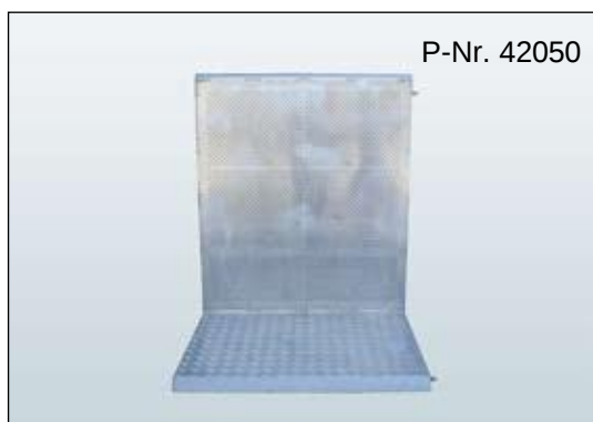
Bühnengitter Typ A · 1,15 x 1,00 m Oberes Rohr Ø: 60 mm, Gewicht: 39,2 kg, Aluminium
