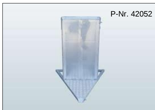
Bühnengitter 45° Vario-Innen Typ A Oberes Rohr Ø: 60 mm, Gewicht: 19,2 kg, Aluminium
