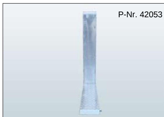
Bühnengitter 22,5° Vario-Außen Typ A Oberes Rohr Ø: 60 mm, Gewicht: 12,8 kg, Aluminium
