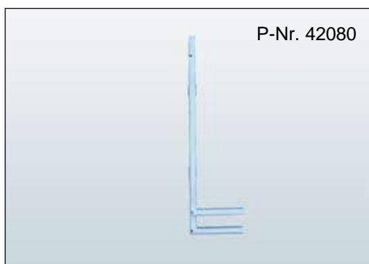
Bühngitter Höhenausgleich Länge: 1150 mm, verstellbar bis Höhe 160 mm, Gewicht: 11,2 kg
