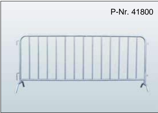
Absperrgitter Typ M - 1,10 x 2,50 m Rohr Außen Ø: 38 mm, Rohr Innen Ø: 22 mm, Gewicht: 22 kg
