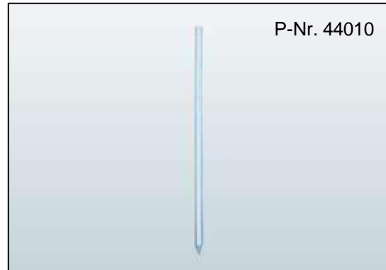
Kunststofffuß Typ K zum Einschlagen für Absperrzaun Typ K, Länge: 1500 mm, Ø 44 mm, Gewicht: 2,2 kg
