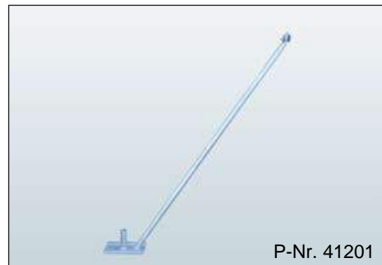
Mobilzaun-Stützstrebe mit Rohr Länge: 1950 mm, Gewicht: 5,9 kg
