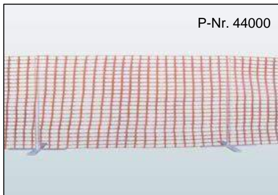
Absperrzaun Typ K 1,00 x 50,00 m PPC-Kunststoff, Farbe orange, Maschenweite 95 x 35 mm, Gewicht: 12,5 kg
